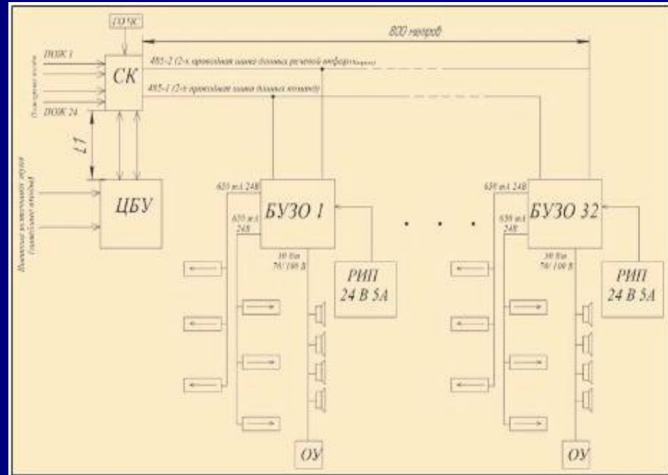
Рис. 1. Распределенная структура системы оповещения
