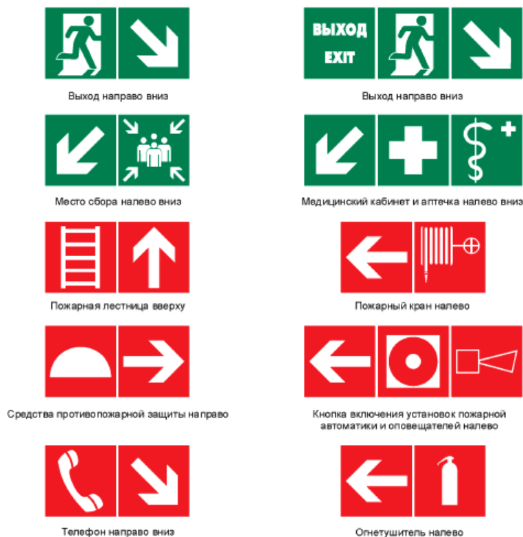
Рисунок 10 - Примеры формирования смысловой комбинации знаков для указания направления движения к эвакуационному выходу, средствам противопожарной защиты, месту сбора и средствам оказания первой медицинской помощи
