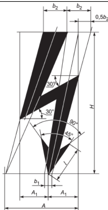
Рисунок Н.1 - Графический символ электрического напряжения
