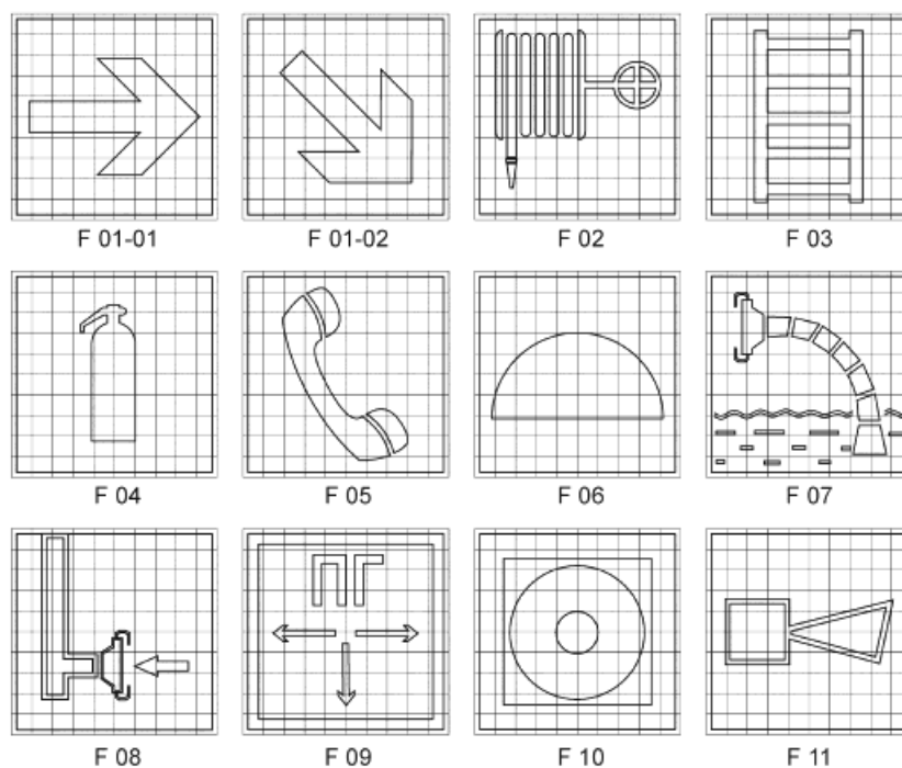
Рисунок П.4 - Знаки пожарной безопасности
