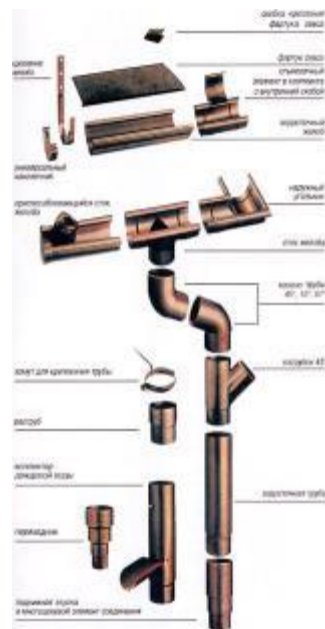
Устройство водосточной трубы с воронкой под водосток
