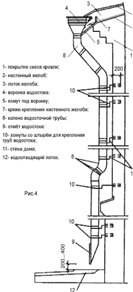
Устройство водосточной трубы с воронкой под водосток
