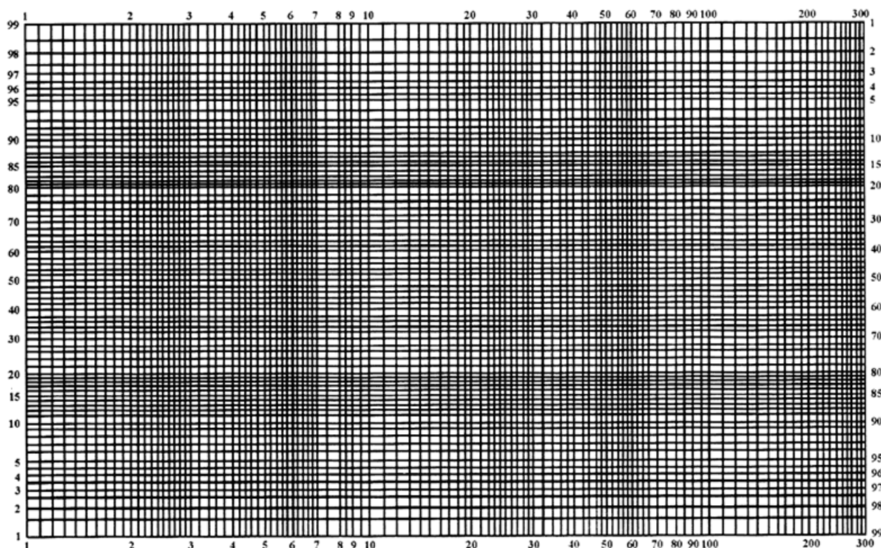
Рис. Логарифмическая вероятностная координатная сетка
