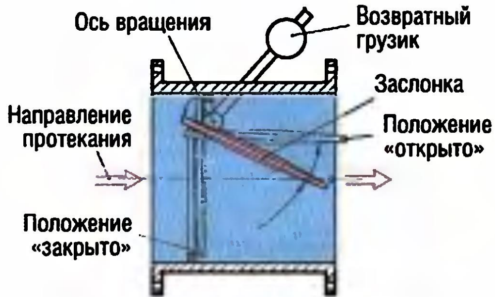
Рис. I.35. Обратная заслонка (с фланцами)
