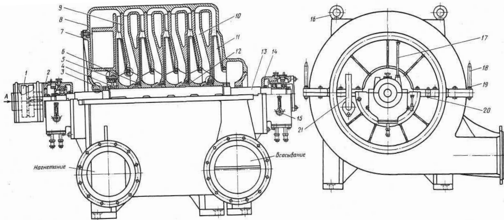
Рисунок 13 – Воздуходувка марки ТВ-80-1,6:
