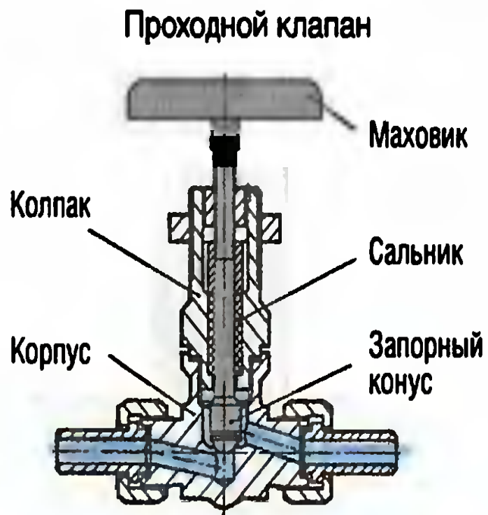
Рис. I.28. Арматура высокого давления
