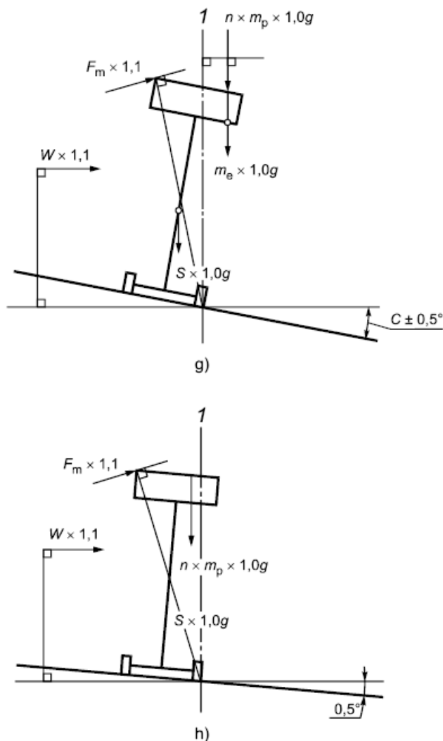
1 - линия опрокидывания; 2 - направление движения; 3 - ограничение вылета; C - максимальный наклон шасси Рисунок 2 - Примеры максимальной опрокидывающей нагрузки и комбинации силового момента
