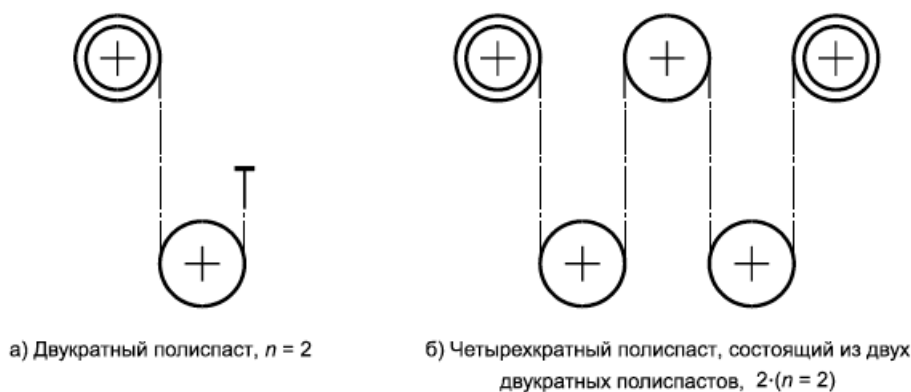
Рисунок С.3 - Полиспасты
