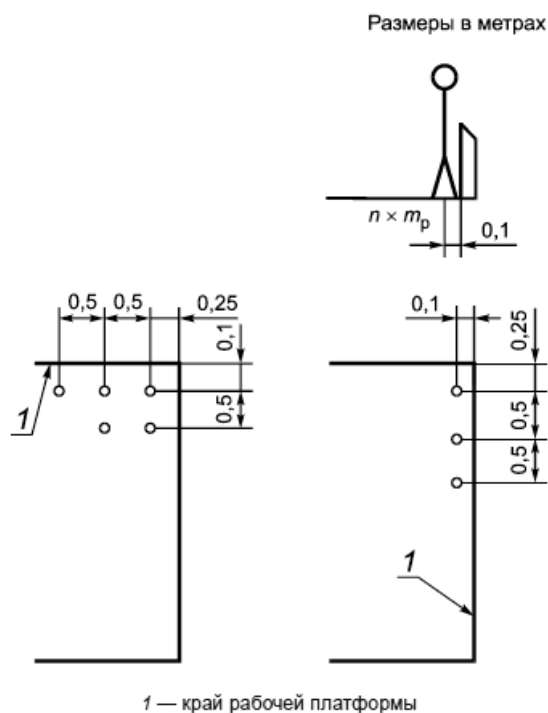
Рисунок 1 - Номинальная нагрузка (масса человека)
