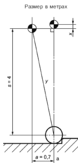
Рисунок Е.2 - Наезд МПП на препятствие
