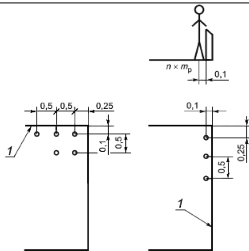
1 - край рабочей платформы
