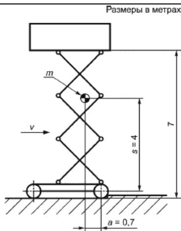
Рисунок Е.1 - МПП перед препятствием
