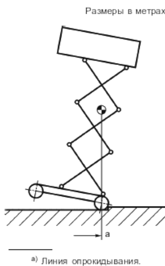
Рисунок Е.2 - Наезд МПП на препятствие
