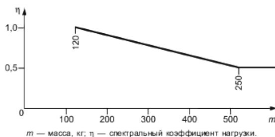
Рисунок 3 - Спектральный коэффициент нагрузки
