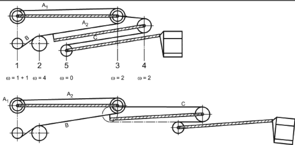
1 - барабан двойного каната; 2 - канатоведущий шкив (отклонение в обратном направлении); 3 - канатоведущий шкив (отклонение в том же самом направлении); 4 - канатоведущий шкив (отклонение в том же самом направлении); 5 - концевое прикрепление каната
