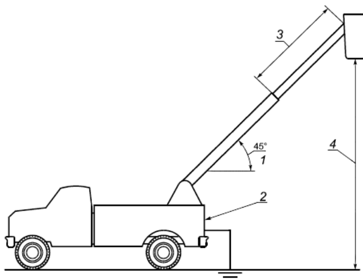
Рисунок 2 - Конфигурация испытания для МПРП с непроводящей (изолирующей) стрелой, оборудованных системой проверки сопротивления заземляющего электрода
