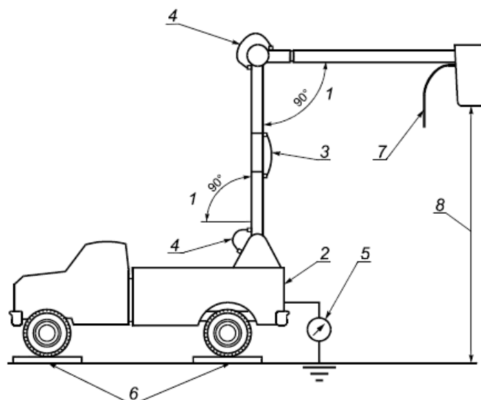
Рисунок 3 - Конфигурация стрелы при проведении испытаний на пробой МПРП с телескопической непроводящей (изолирующей) стрелой
