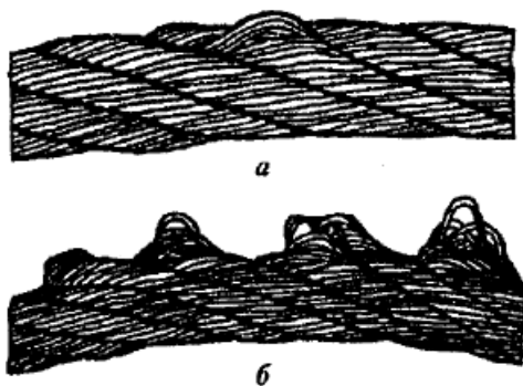
Рисунок 12. Выдавливание проволок прядей:
