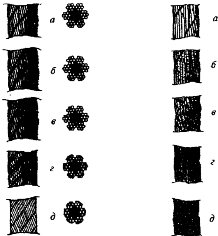
Рисунок 5. Износ наружных проволок каната крестовой свивки:
