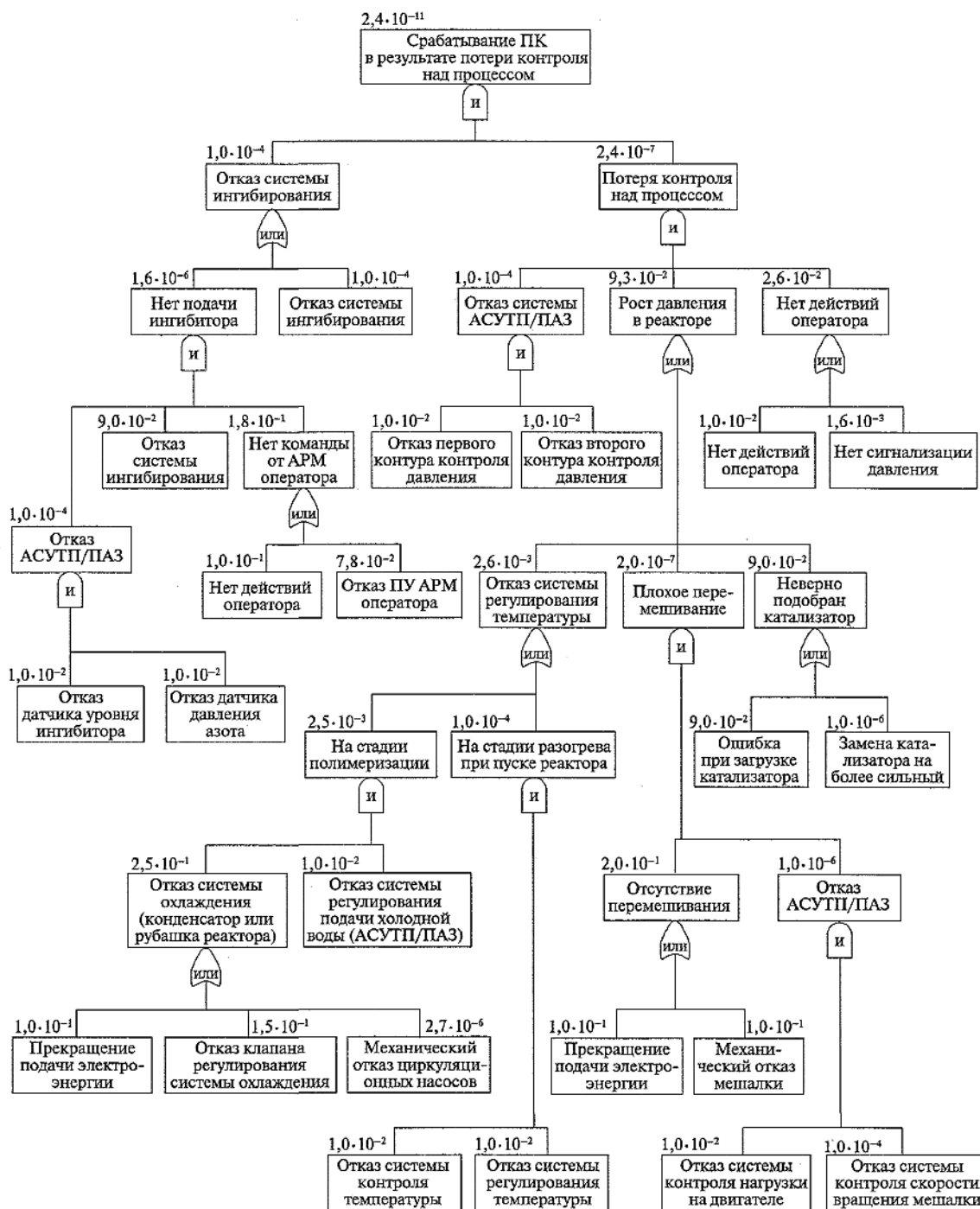
Рисунок 8-1. Пример дерева отказов для химических реакторов
