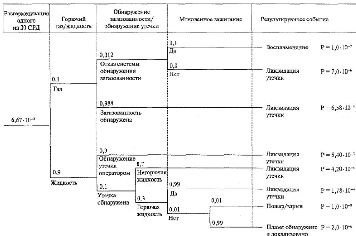
Рисунок 8-2. Пример дерева событий для случая разгерметизации сосудов, работающих под давлением
