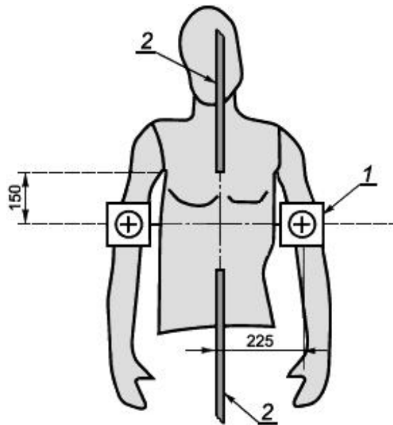
Рисунок 5 - Шина электропитания и электродуговые электроды относительно положения(ий) манекена(ов)
