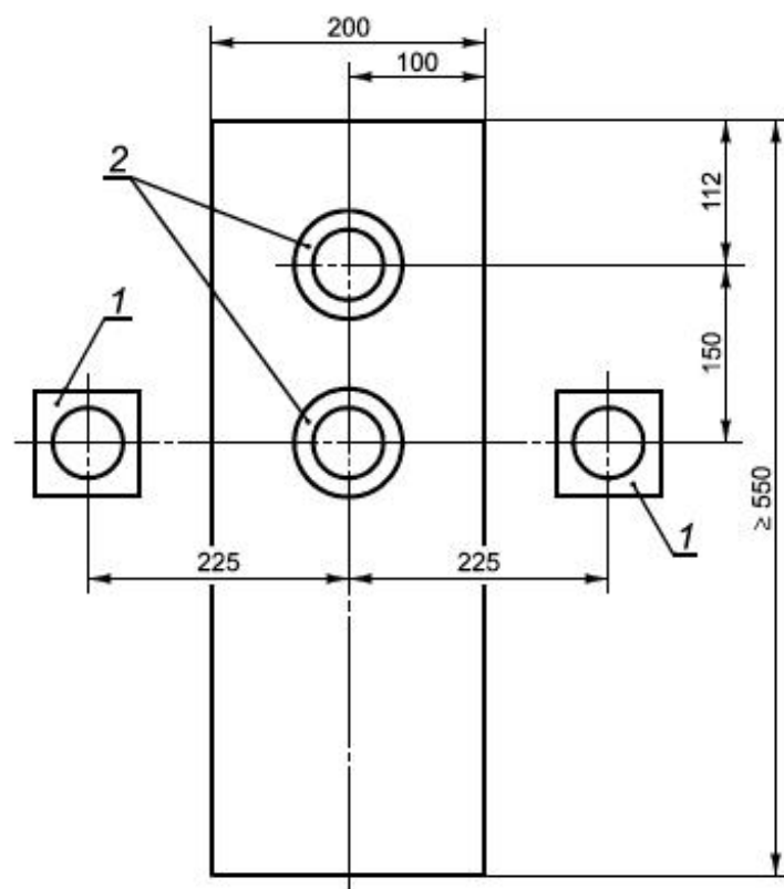
1 - контрольные датчики; 2 - датчики, вмонтированные в панель
