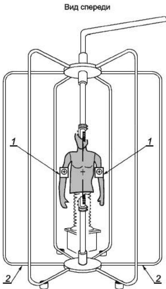
Рисунок 4 - Метод А: Подвижная панель с двумя датчиками
