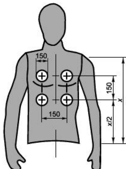
Рисунок 6 - Расположение электродов и контрольных датчиков
