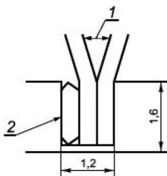
а) Установка термопары в калориметре
