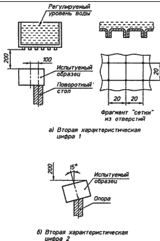
Рисунок 3 - Устройство для проверки защиты от вертикально падающих капель воды (емкость для получения капель)
